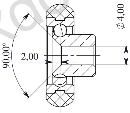
SEZIONE A-A
