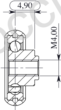
SEZIONE A-A
