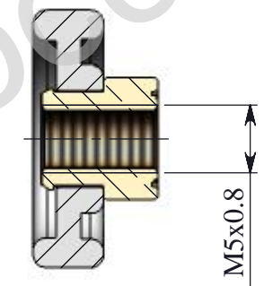
SEZIONE A-A
