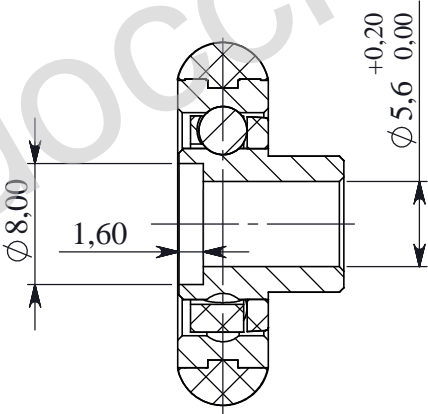
SEZIONE A-A
