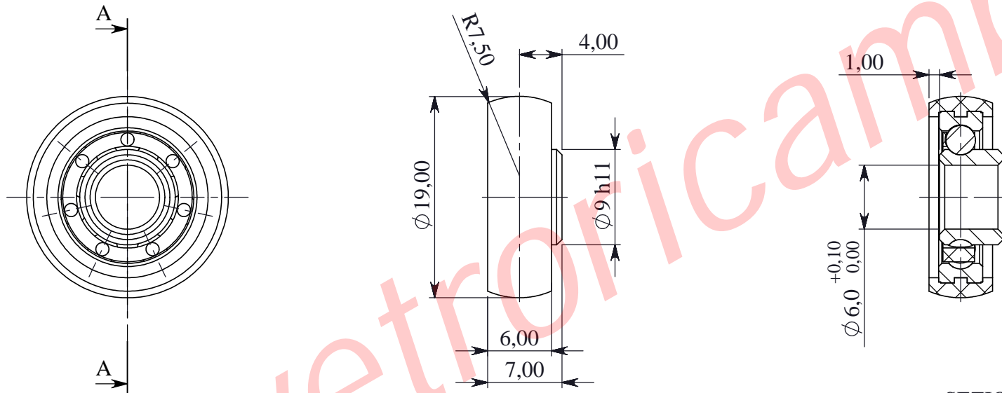
SEZIONE A-A
